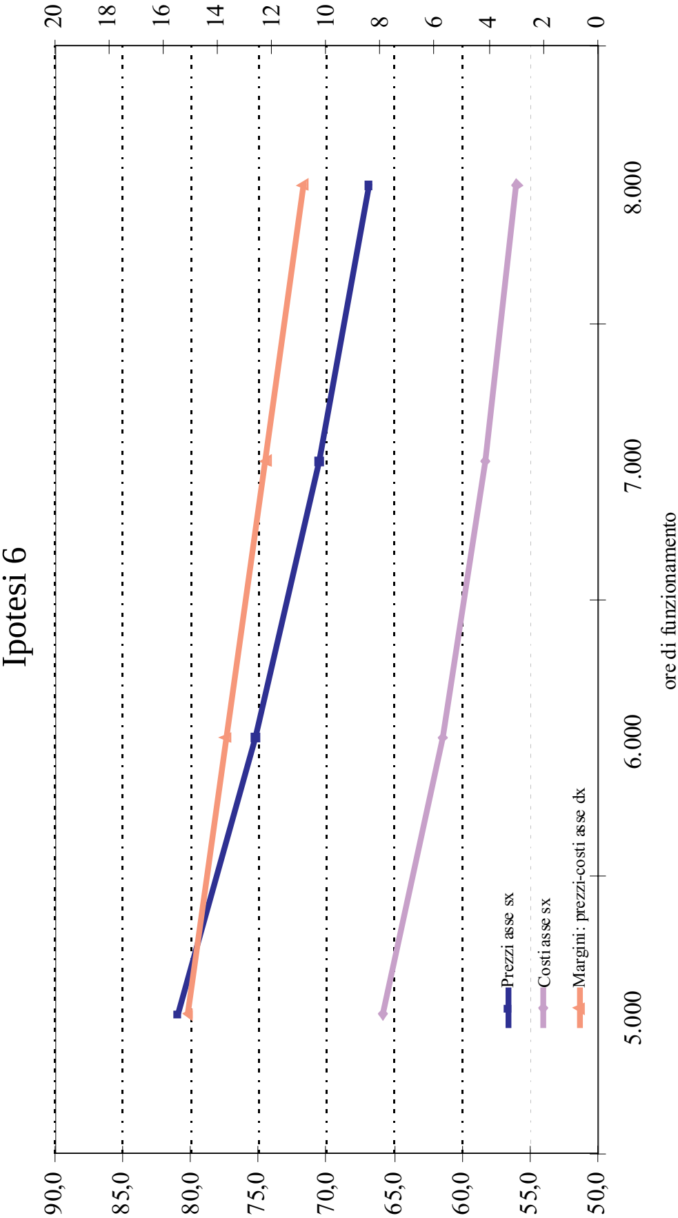
Fig. 2.2.1.6 SER: prezzi e costi dell'elettricità al 2008 in funzione delle ore di funzionamento (£/kWh)
